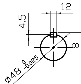
B 矢視図
