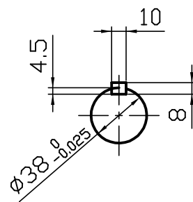
B 矢視図
