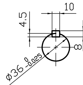
C 矢視図
